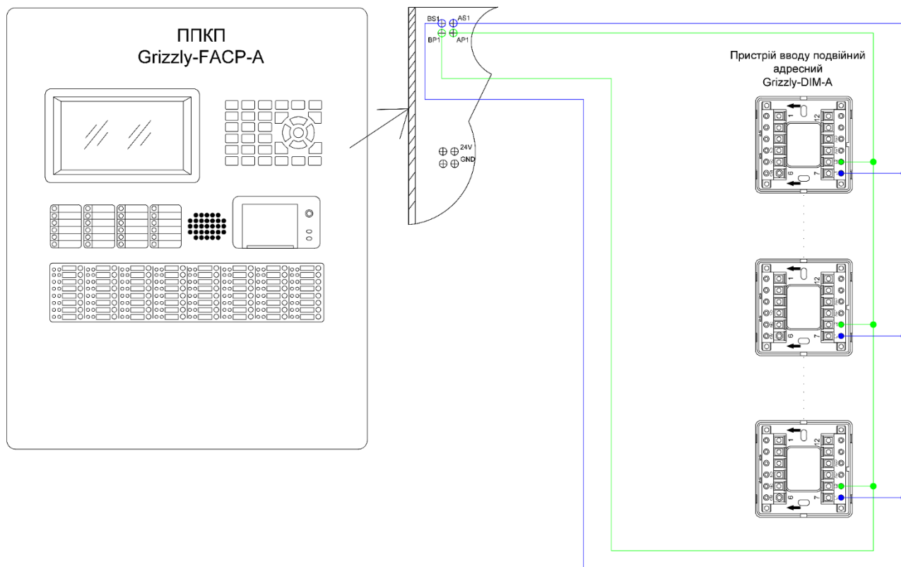
Рисунок 4 – Приклад підімкнення пристрою до ППКП
