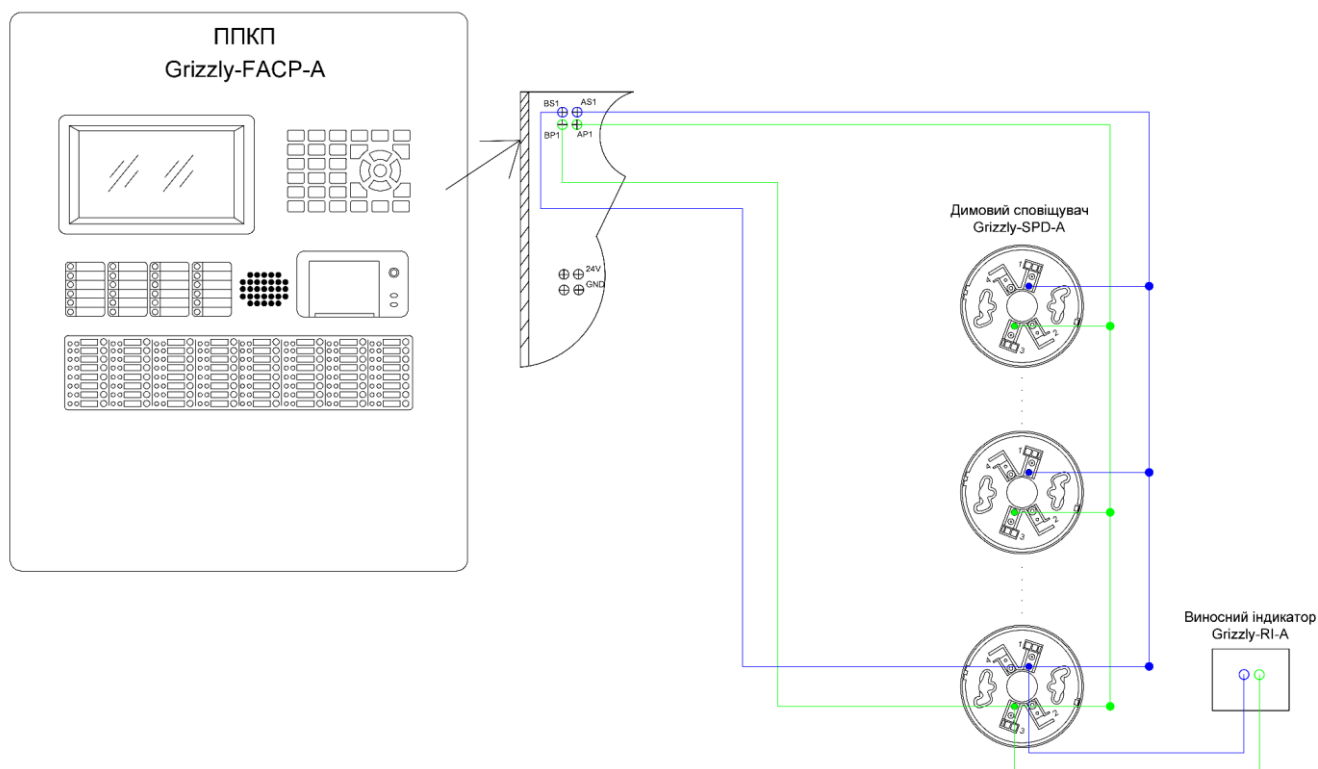
Рисунок 4 – Схема підімкнення сповіщувачів до ППКП
