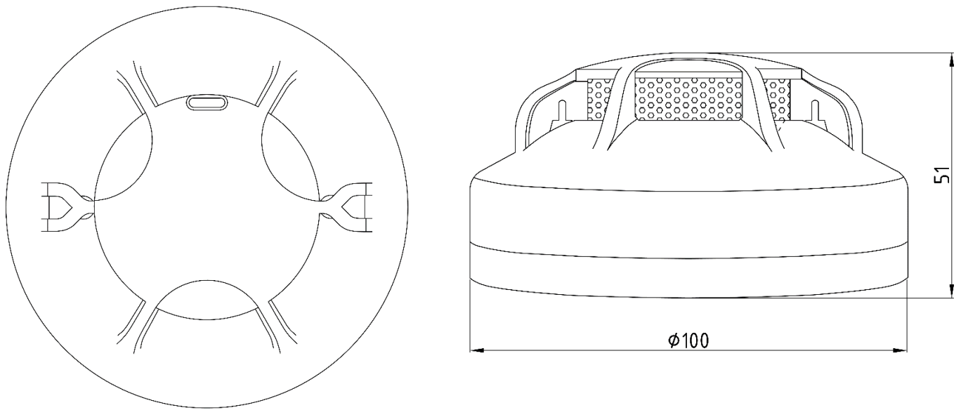
Рисунок 1 – Загальний вигляд сповіщувача зверху (ліворуч) та збоку (праворуч)
