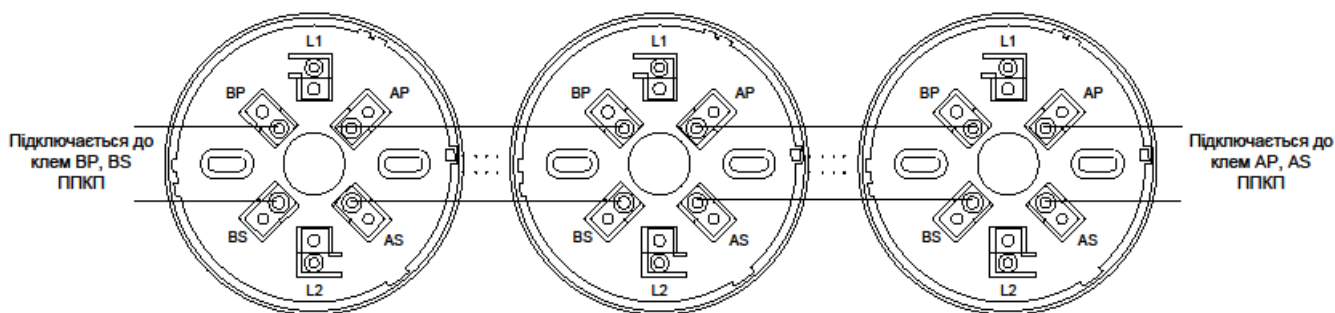
Рисунок 5 – Схема підімкнення баз Grizzly-IB-A до ППКП
