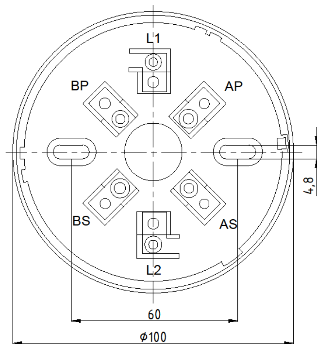
Рисунок 3 – Загальний вигляд бази Grizzly-IB-A
